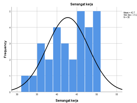
Gambar 1 Histogram Variabel Semangat Kerja (X)
